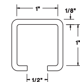
GUIDE RAIL: 191007
